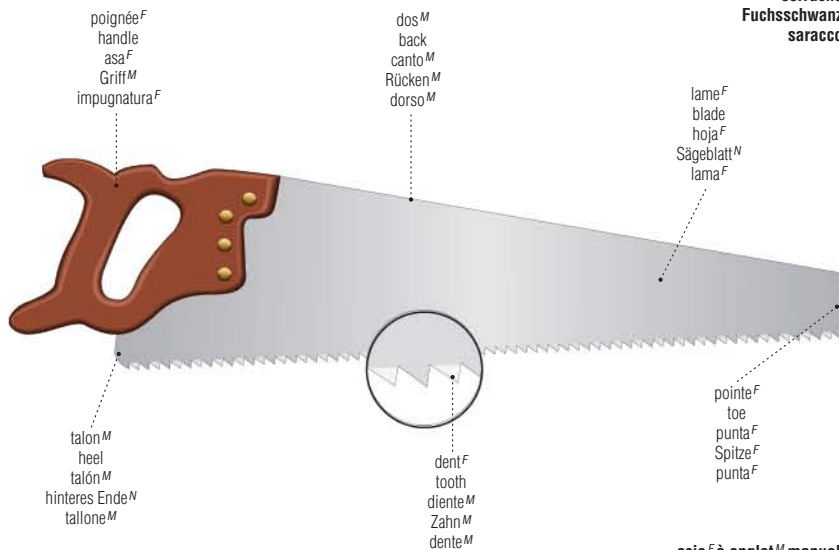
scie F à onglet M manuelle hand miter saw sierra F de ingletes M Hand-Gehrungssäge F sega F per agnatura F manuale
